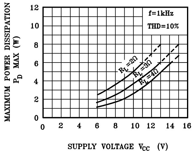
P D MAX - V CC
